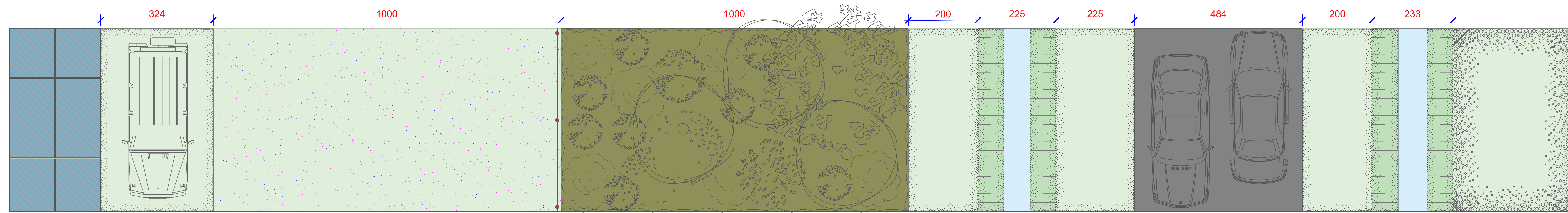
Zonnepanelenopstelling Graspad Bloem- & kruidrijk grasland Hekwerk Groenstrook / struweel Onderhoudspad Zaksloot Berm Openbare weg Riethmsteeg Berm Zaksloot Wei-/grasland / akker
